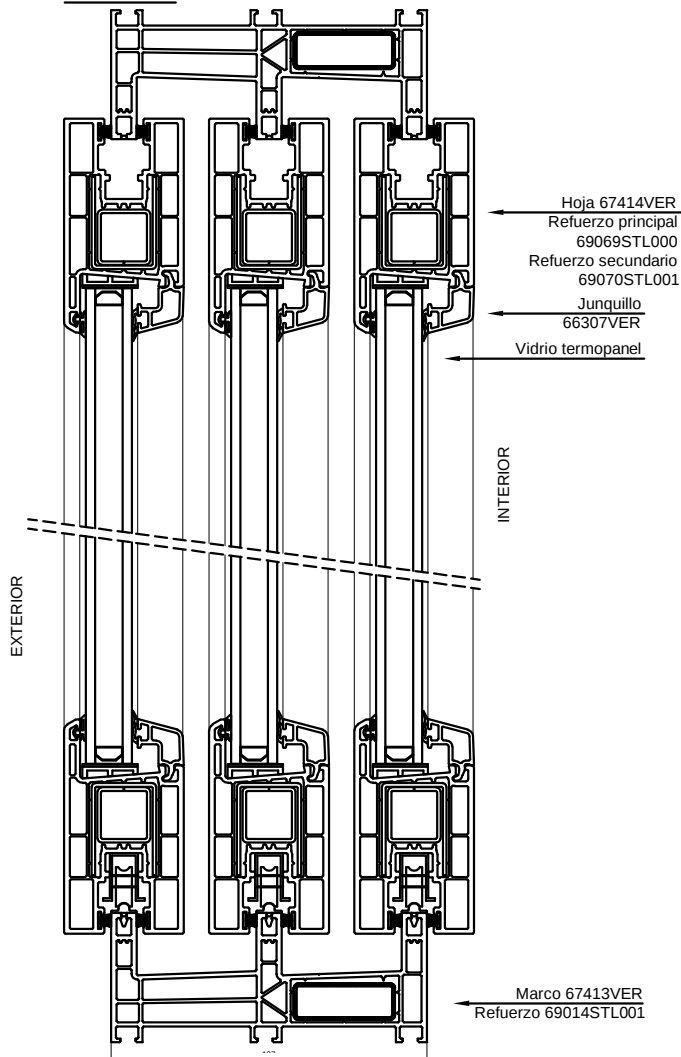
DETALLE 2
