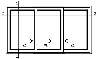
DETALLE 1
