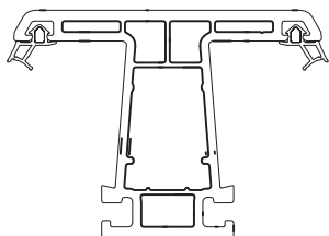
Barra T corredera 7416
