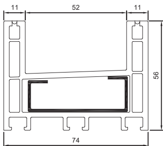
Marco corredera 2 hojas 7401
