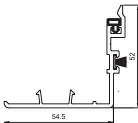
Hoja corredera chica 7415
