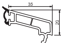
Junquillo para vidrio 4mm 6306
