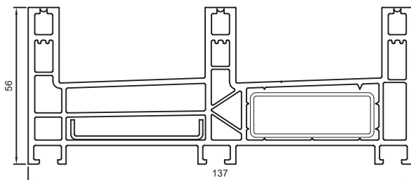
Marco corredera 3 hojas 7413
