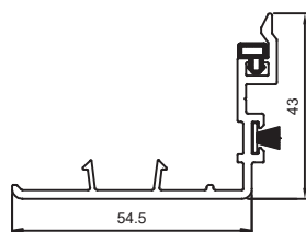
Traslapo hoja corredera chica 7419
