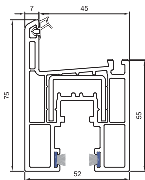
Hoja corredera chica 7415
