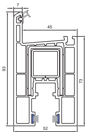
Hoja corredera grande 7414
